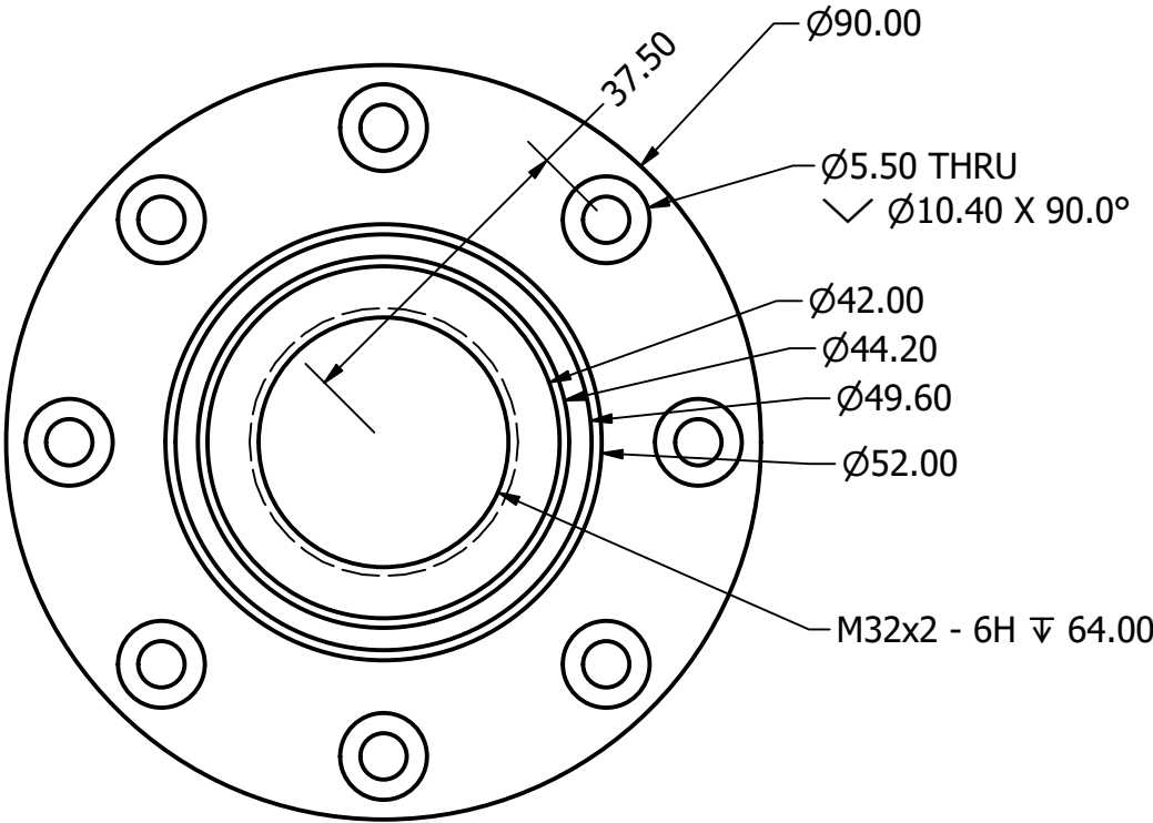
BOTTOM SCALE 1 : 1
